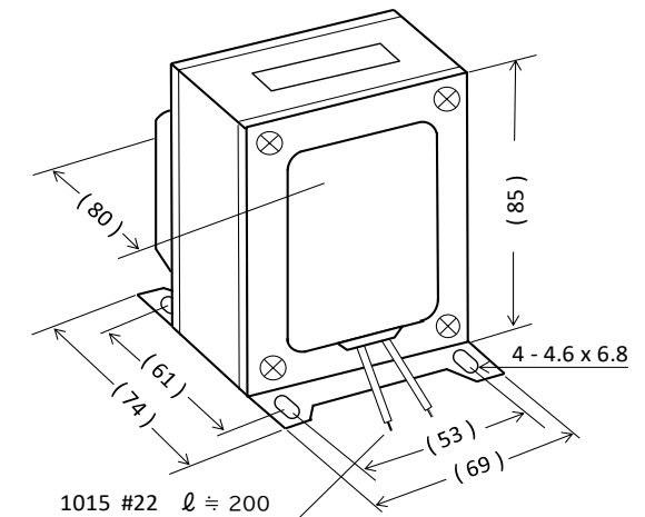
外形寸法図 コアリング付き
