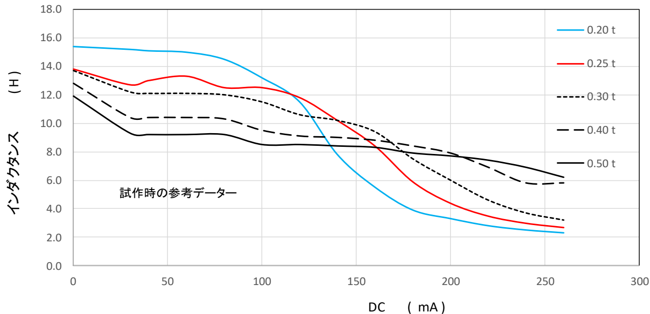
同じ巻き数でもコアギャップの値によりL値が変わります
