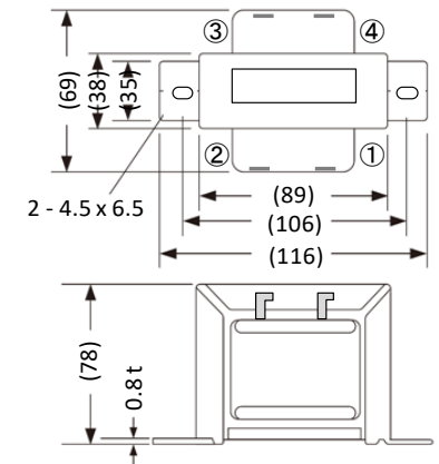
外形寸法図
