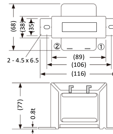
外形寸法図
