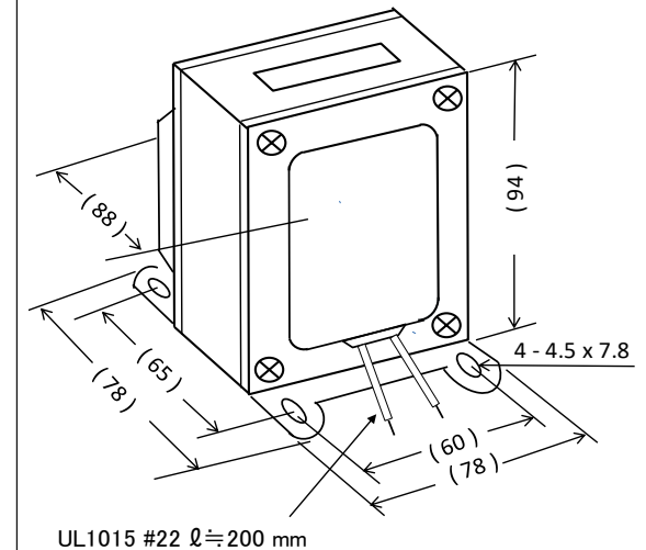
外形寸法図
