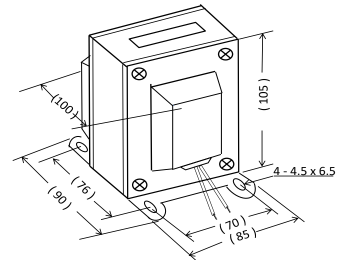
外形寸法図
