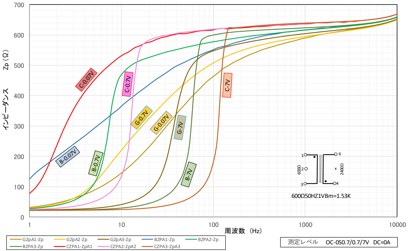
A24-24K06 GBC (A巻き) Level特性比較
