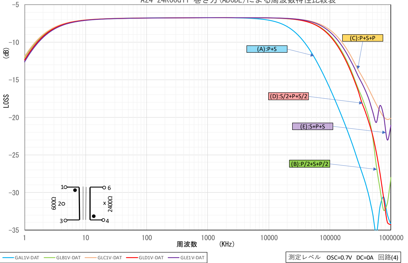
A24-24K06G11 巻き方(ABCDE)による周波数特性比較表
