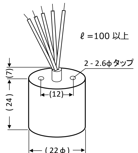
外形寸法図
