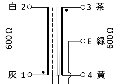
接続図
