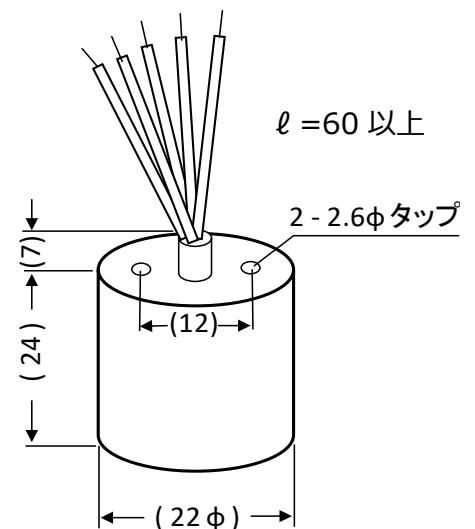
外形寸法図
