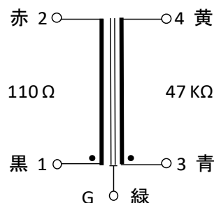
接続図
