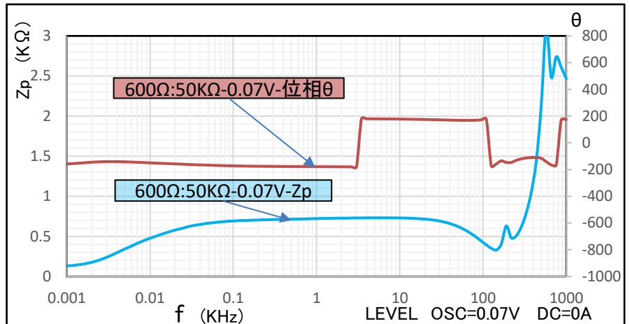
MCL-06K50B NO1 (0.1Vpp) 一次インピーダンス特性表
