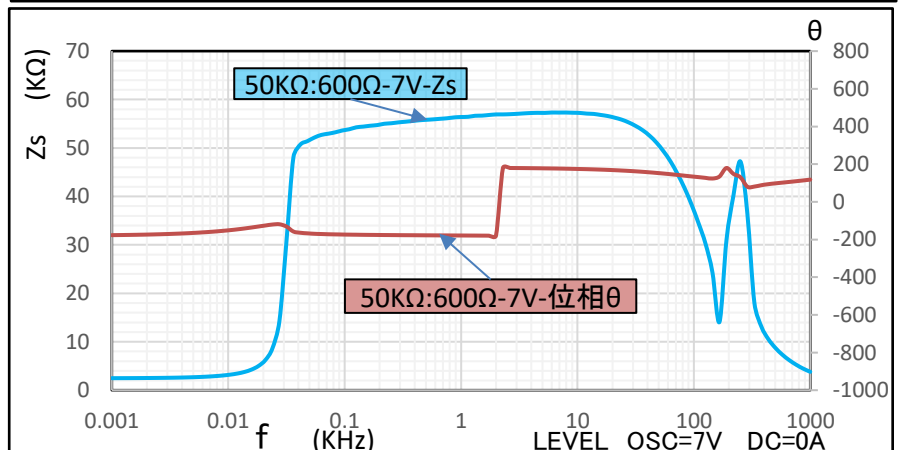
MCL-06K50B NO1 (10Vpp) 二次インピーダンス特性表
