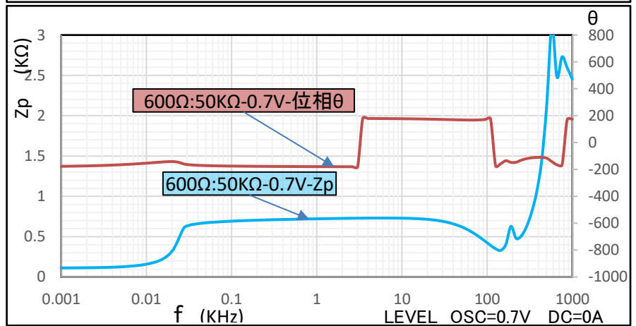
MCL-06K50B NO1 (1Vpp) 一次インピーダンス特性表
