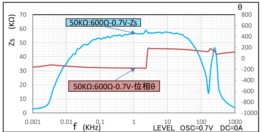
MCL-06K50B NO1 (1Vpp) 二次インピーダンス特性表
