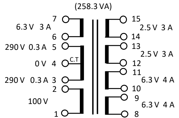
F・R 端子
