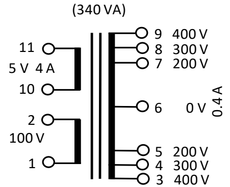
F・R 端子
