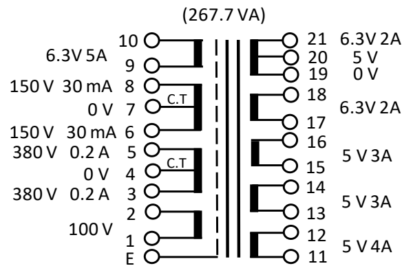
F・R 端子
