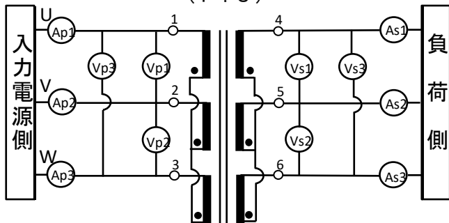
(1) EC型 Y:Y (P : S)
