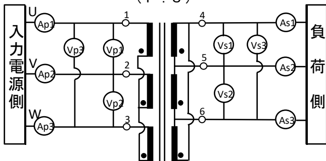
(3) EC型 Y:Δ (P : S)
