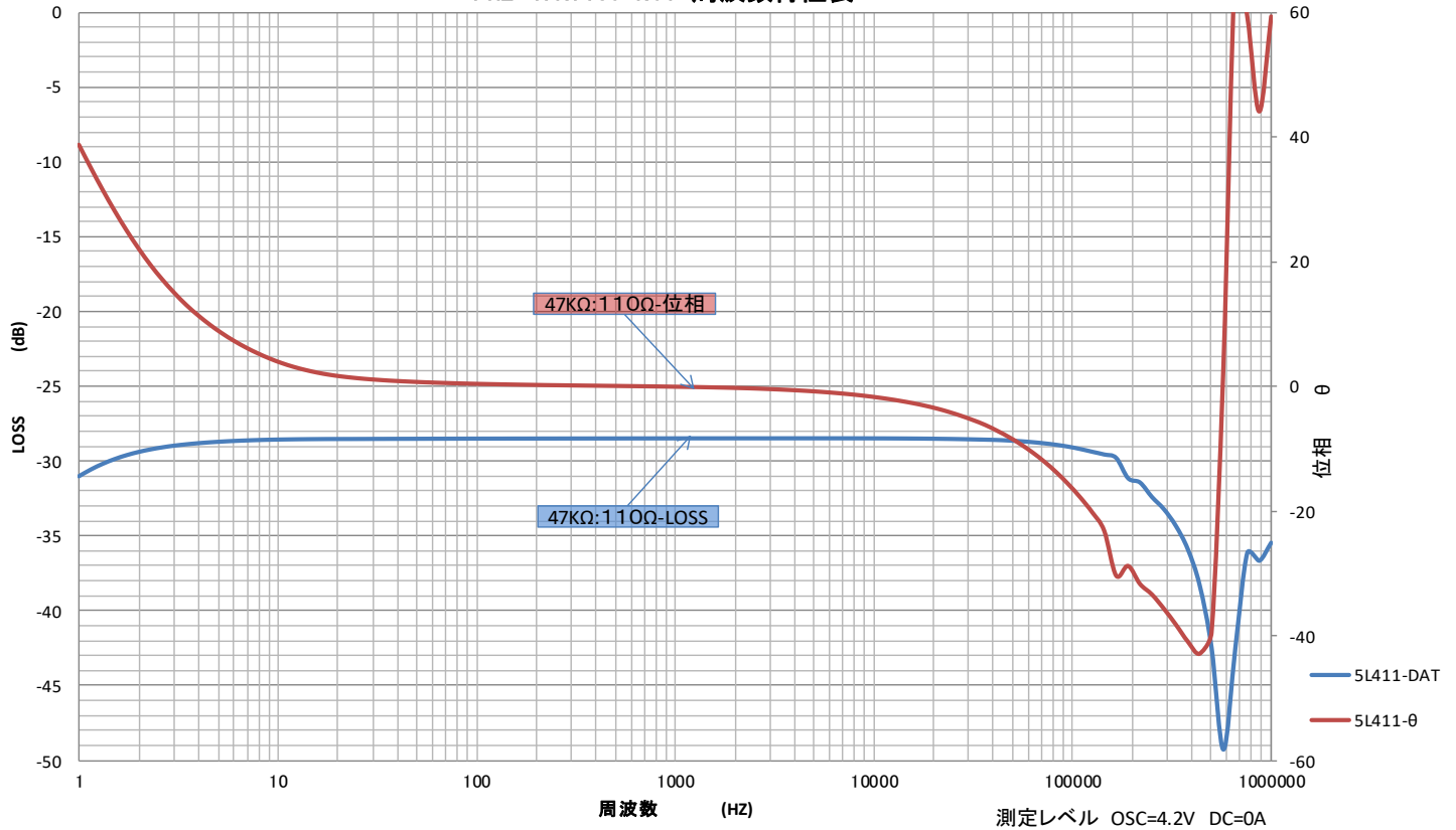
PHL-47K11S5 N01 周波数特性表
