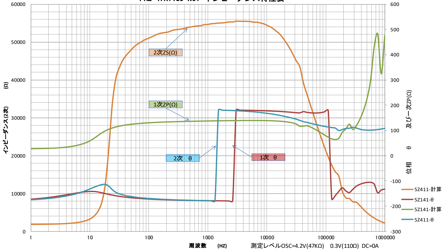
PHL-47K11S5 N01 インピーダンス特性表
