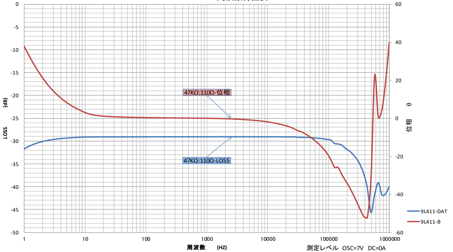
PHL-47K11S9 N01 周波数特性表
