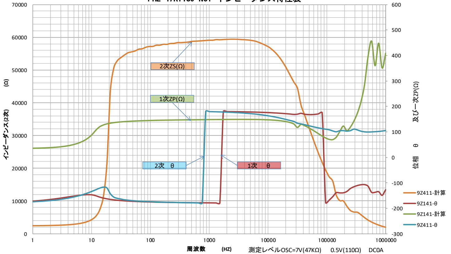
PHL-47K11S9 N01 インピーダンス特性表
