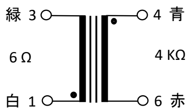
接続図
