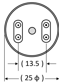
外形寸法図
