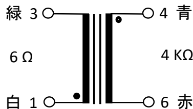
接続図
