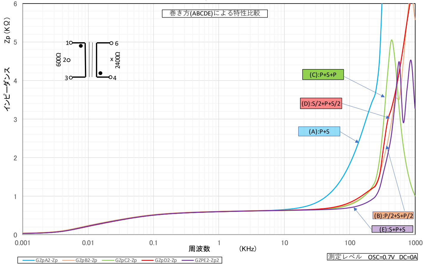
A24-24K06G11 Z p インピーダンス特性表
