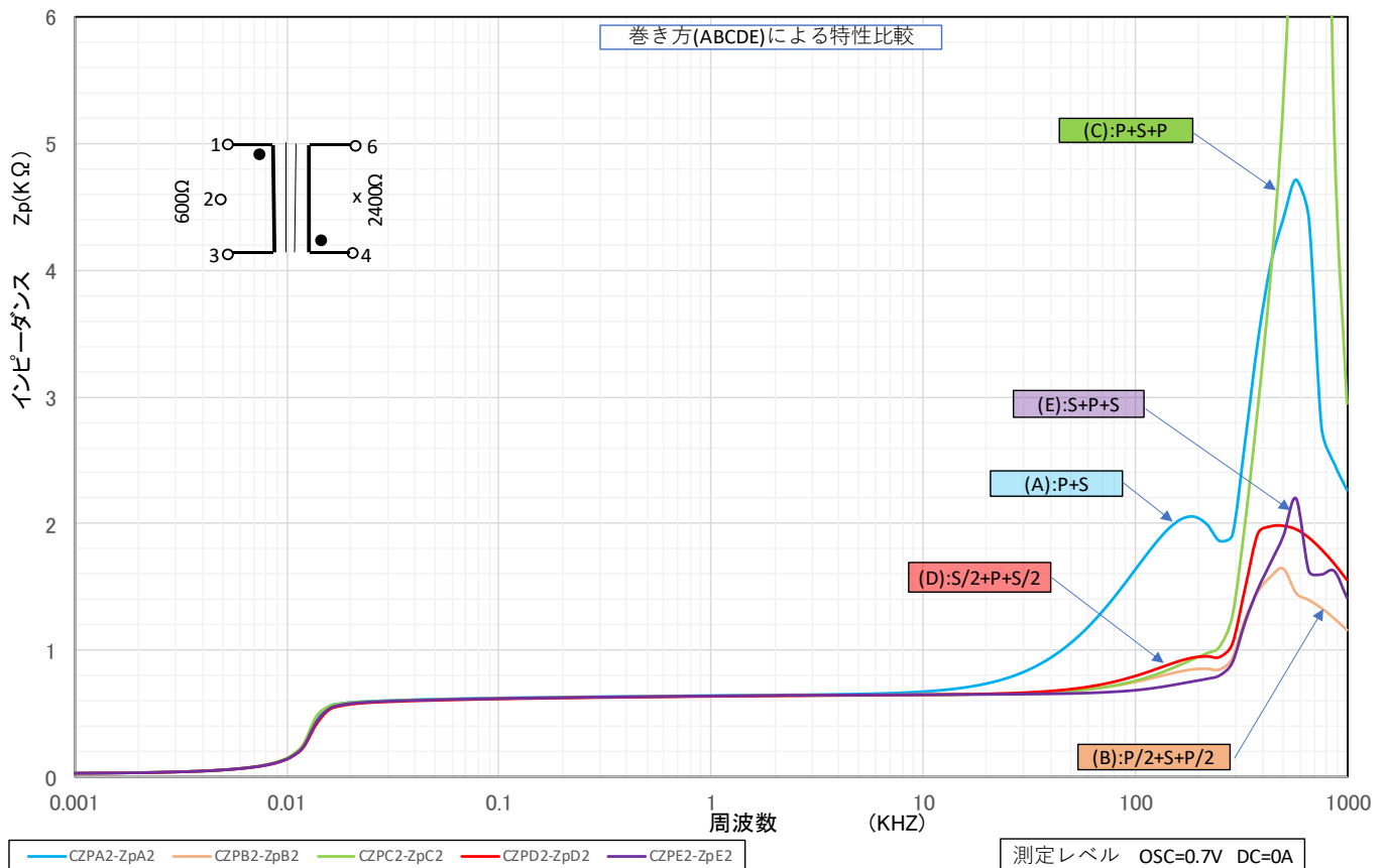
A24-24K06PC Zp インピーダンス特性表
