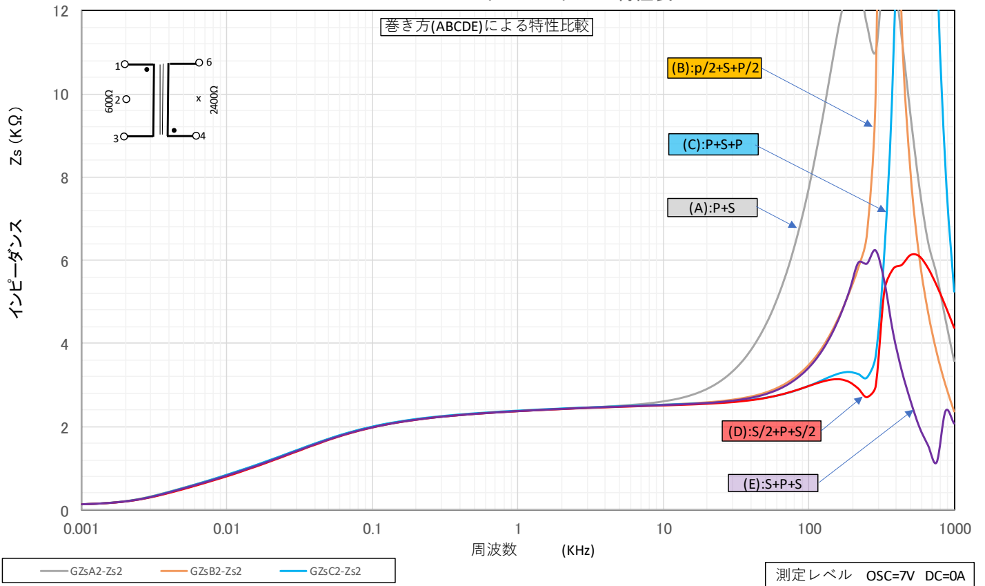
A24-24K06G11 Zsインピーダンス特性表
