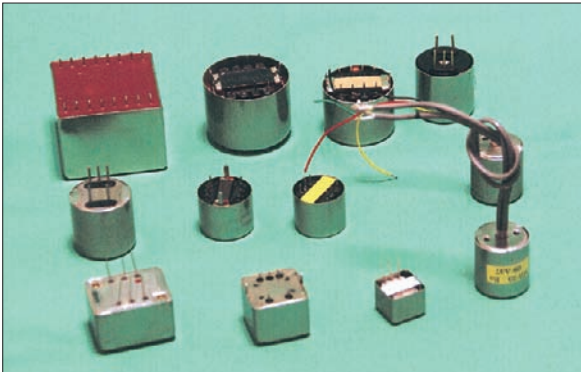
59) PC ケース入りトランス
