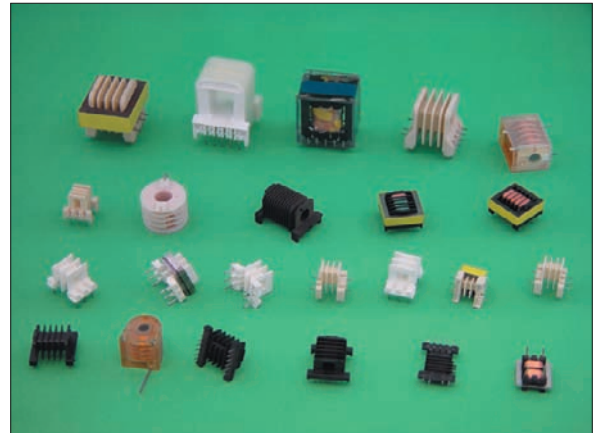
38) 高圧コイルトランス
