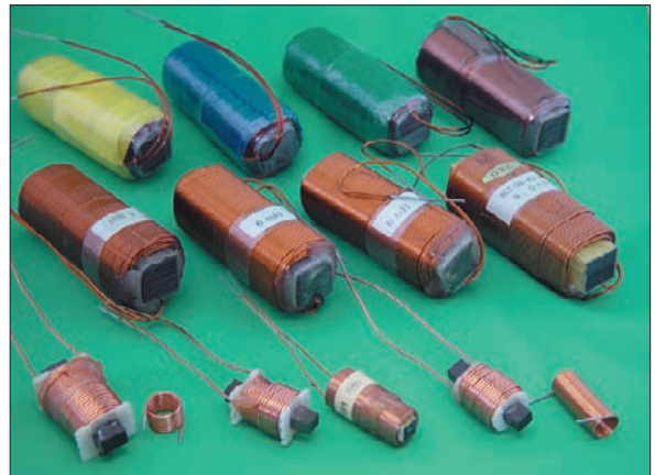
48) ネットワークコイル
