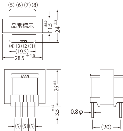
(A) : P28M 外形図
