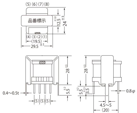
(B) : P28MK 外形図
