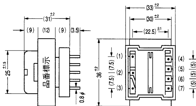
外形図
