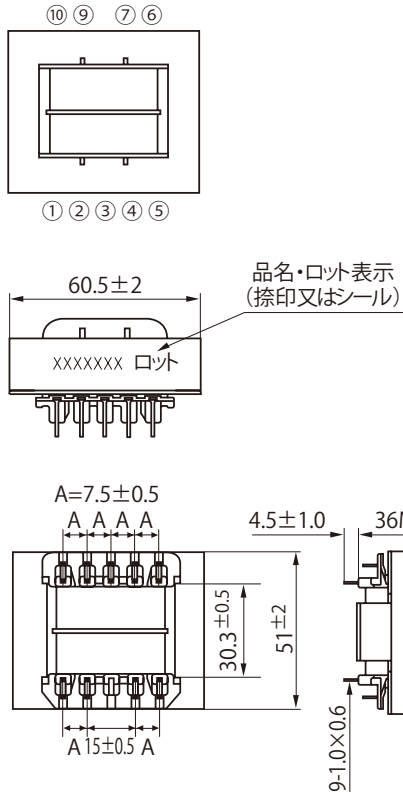
(3) P616K 外形図
