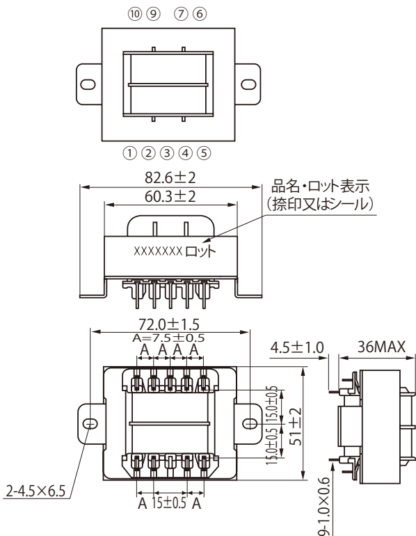
(3) P616K 外形図
