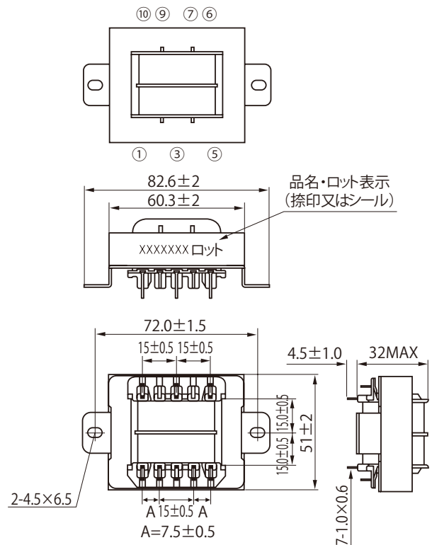
(4) P613K 外形図
