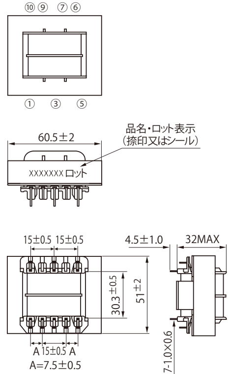
(2) P613 外形図
