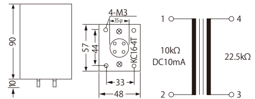
KC16-4T
