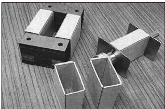
(5) U型用巻芯の例
