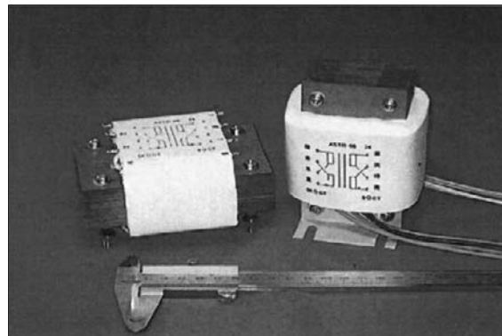
(2) ASTR-06, ASTR-06L の例
