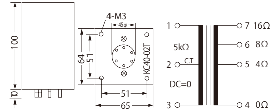
KC40-02T
