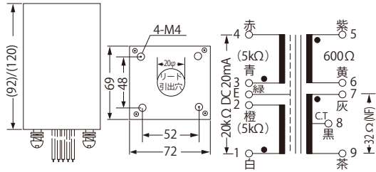
A60-38 DRV
