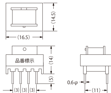
外形図：FT16 (2-17)
