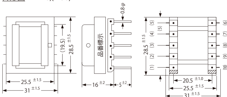
外形図：AL28,(2-36)
