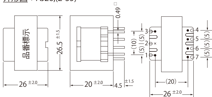
外形図：AJ26,(2-35)
