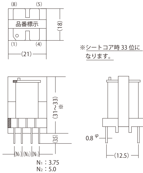
外形図：FTL19,(2-26)
