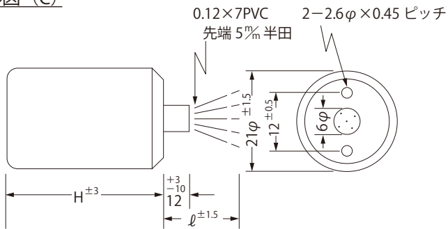
外形図 (C)
