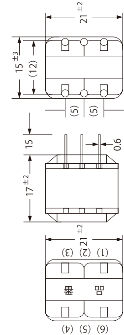
外形図 (2) L16 型
