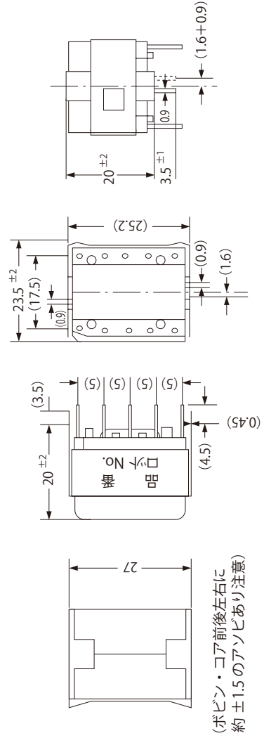
外形図 (1) EP20 型
