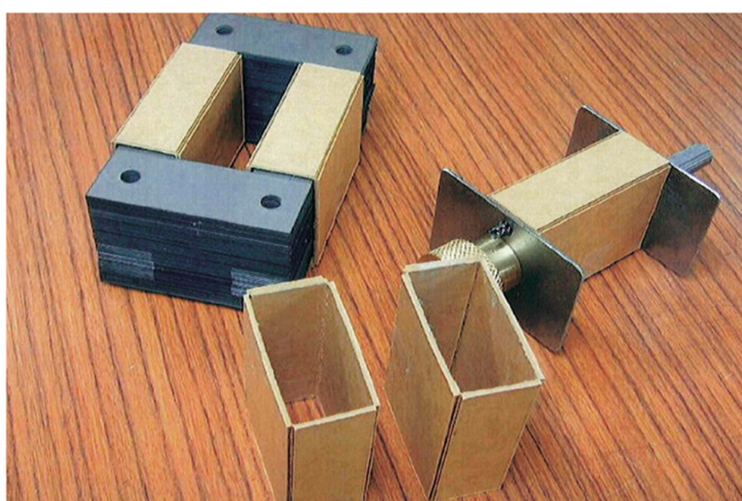
(5)U型用巻芯の例
