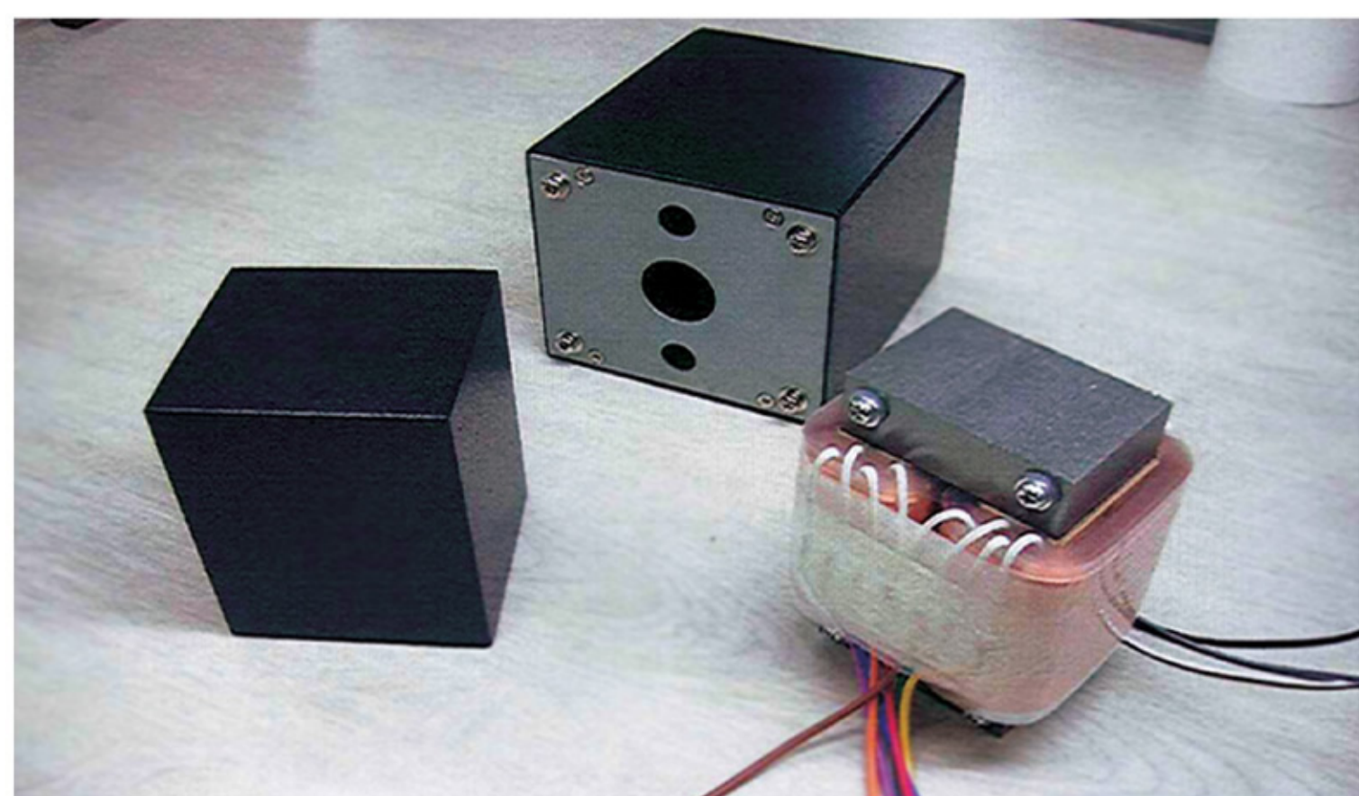
(7)U型のコイルとケースの例
