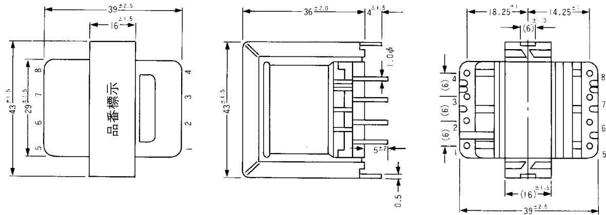
PT4114PE型
