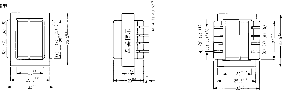
AS-3510A型
