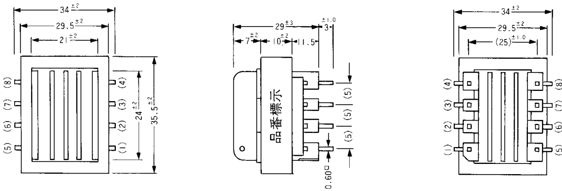
PT4114PE型
