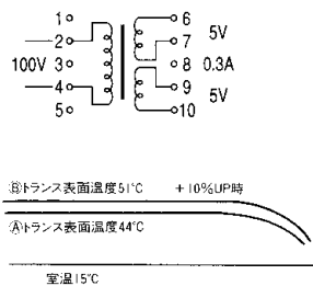
① P48-246U電源トランス
