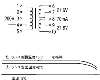
② P48-91U電源トランス
