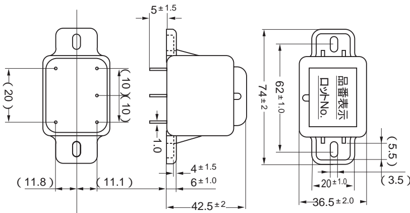
外觀寸法図
