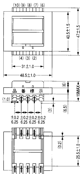
1) 外観寸法図
