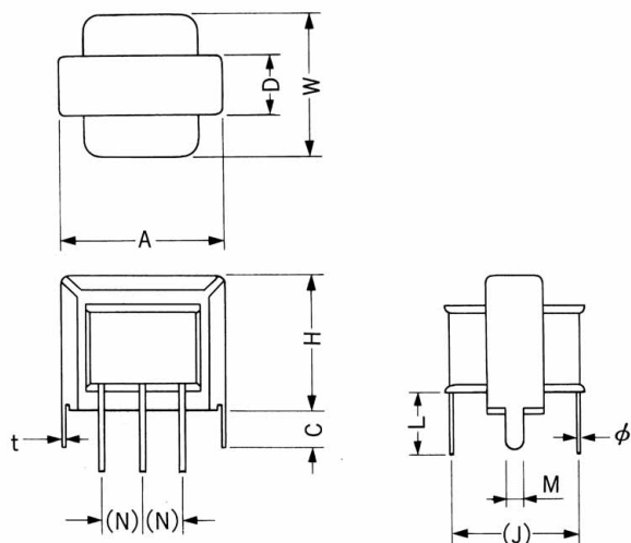
〔外形寸法図〕
